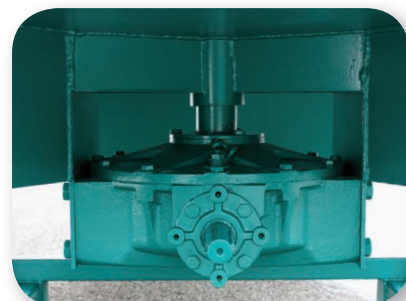
Boîtier de transmission avec renvoi d'angle
