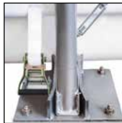
Fixation de la bâche sur la platine des pieds
